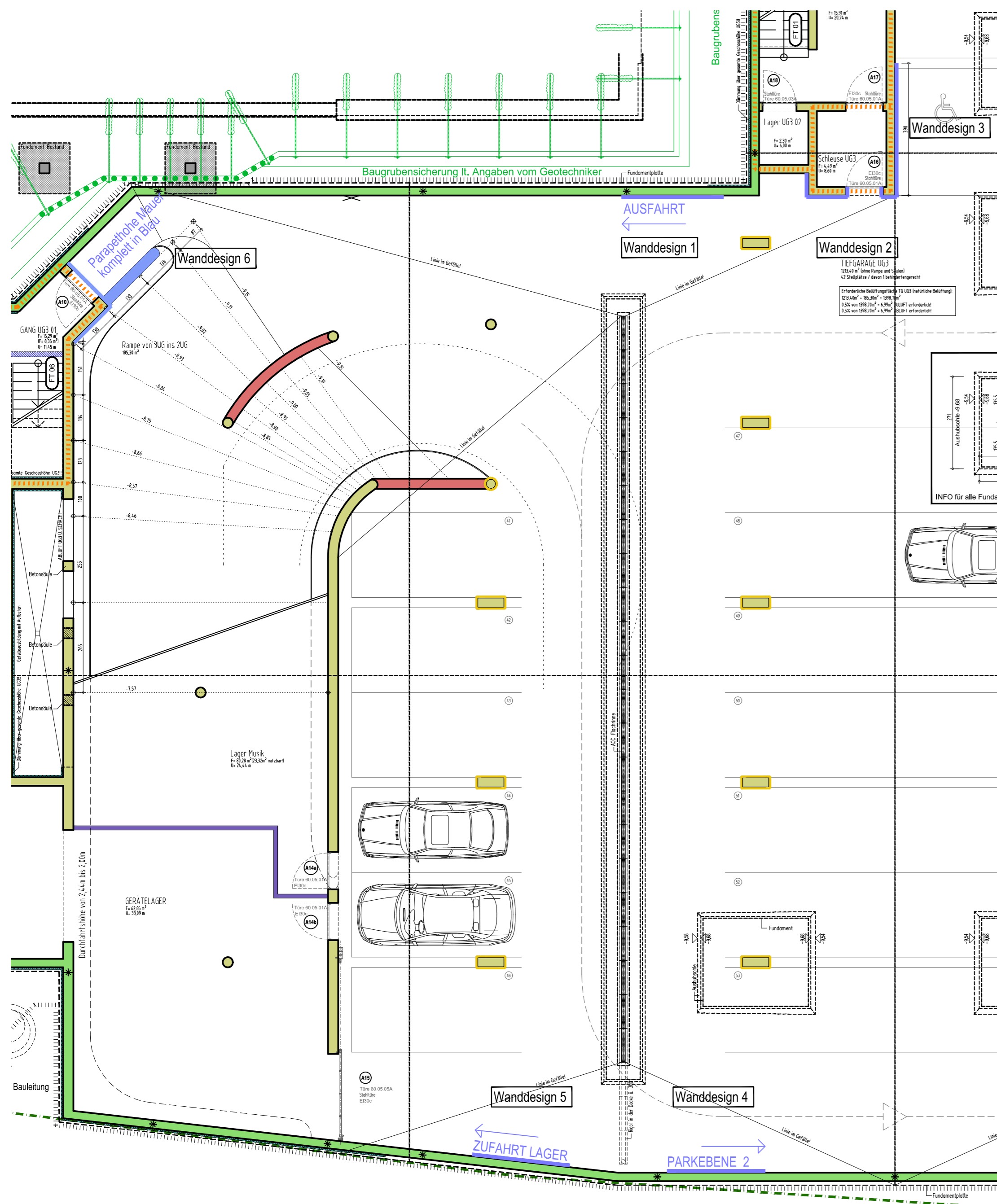
Übersichtsplan Grundriss UG3 M1:100
