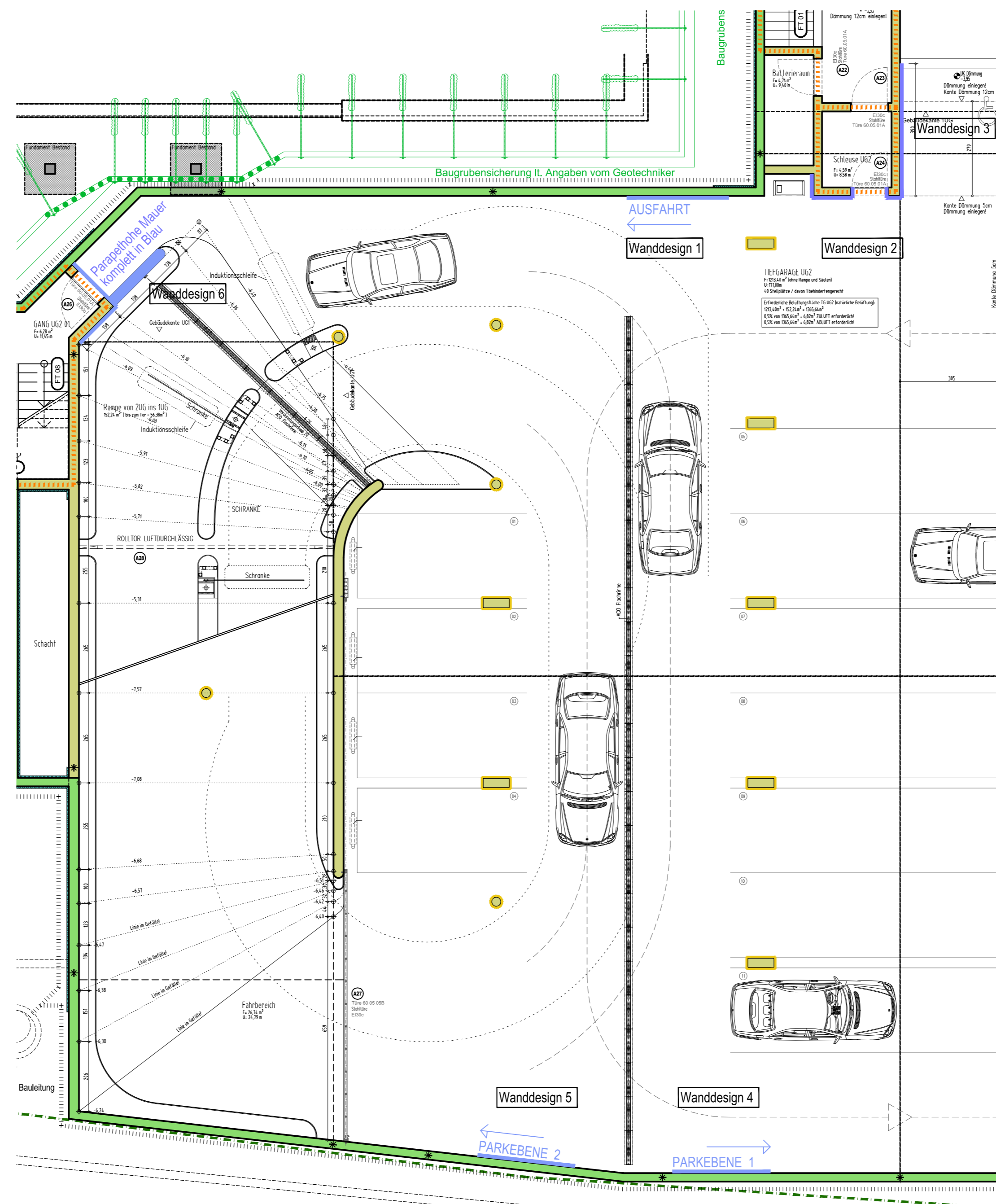
Übersichtsplan Grundriss UG2 M1:100
